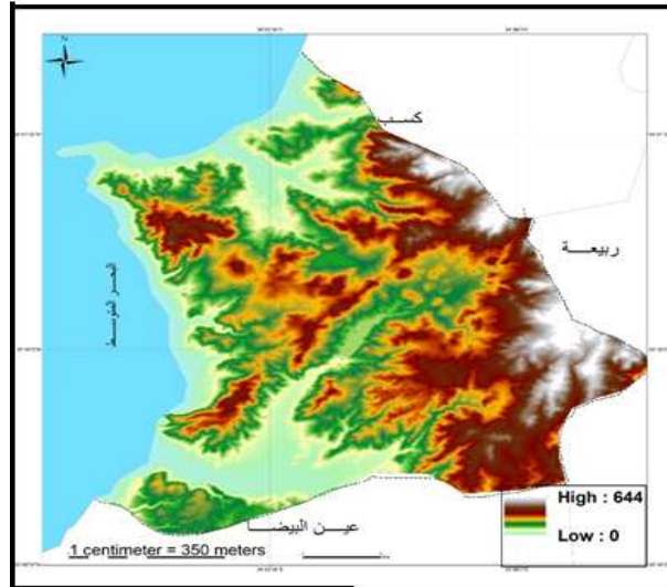
الخريطة (2) نموذج الارتفاع الرقمي (DEM) لناحية قسطل معاف.
