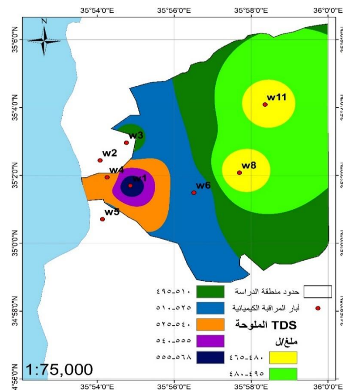
الشكل (3) تغيرات الملوحة في منطقة الدراسة
