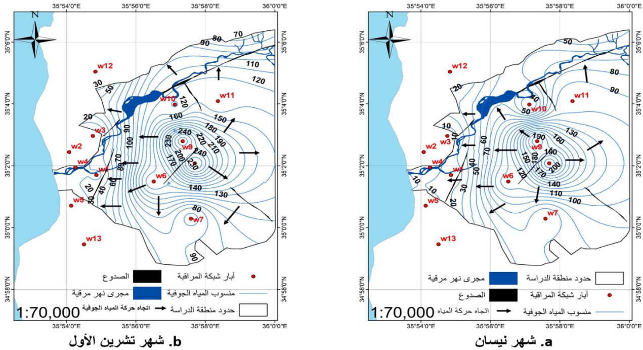
الشكل (4) خارطة هيدرونياميكية في منطقة الدراسة
