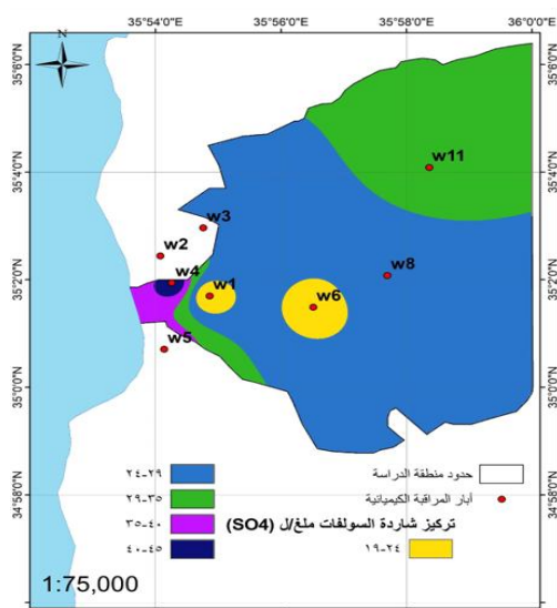
الشكل (6) توزيع الشوارد السالبة في منطقة الدراسة ( القيم مأخوذة وسطياً لفترتي التحليل الكيميائي).
