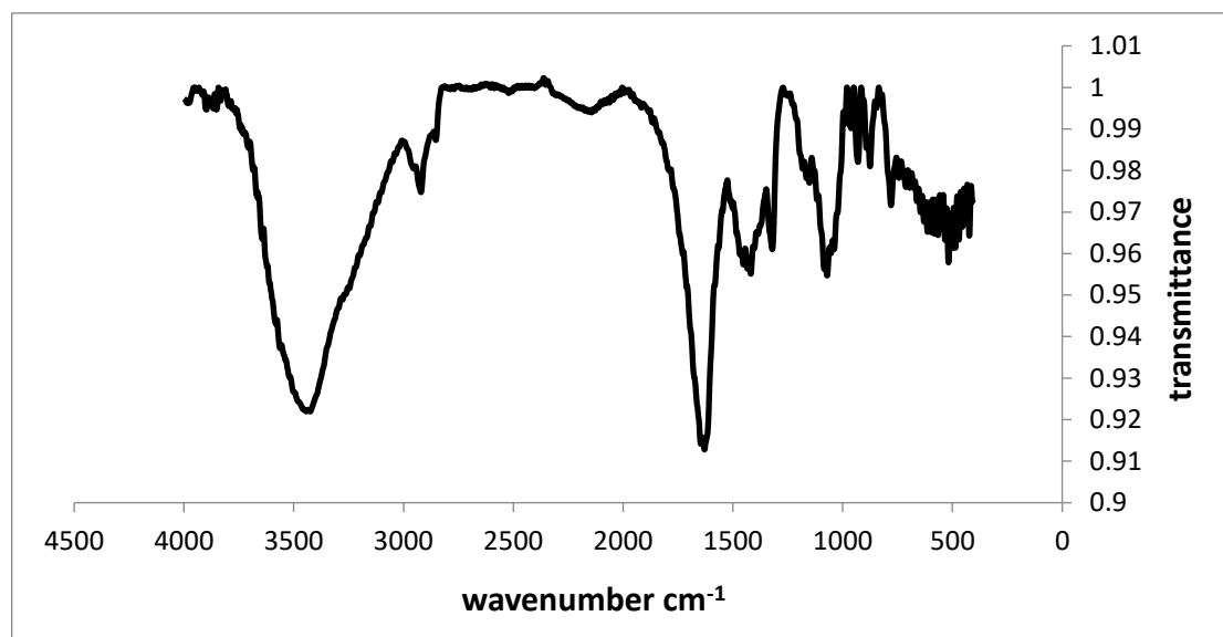
الشكل 6: طيف FTIR لجزيء PHB المستخلص من زهرة النيل
