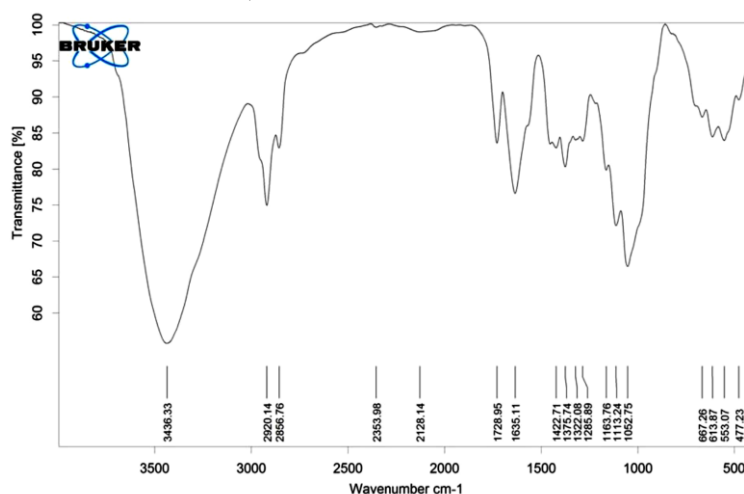
الشكل 7: طيف FTIR لجزيء PHB مرجعي (Preethi et al. , 2015)
